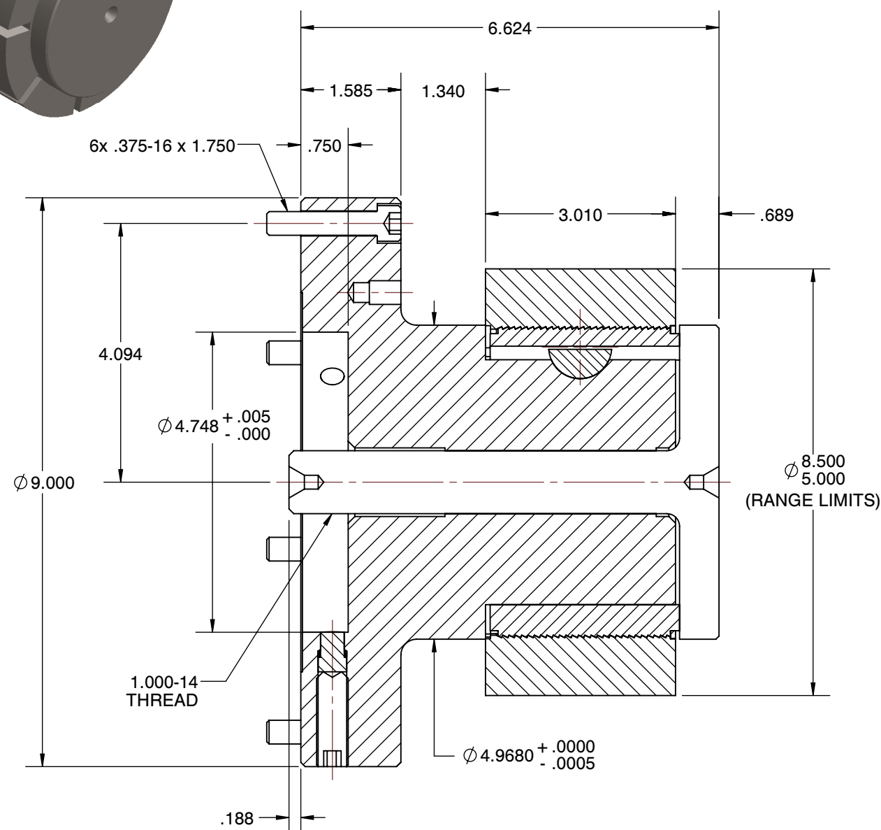
SECTION A-A
