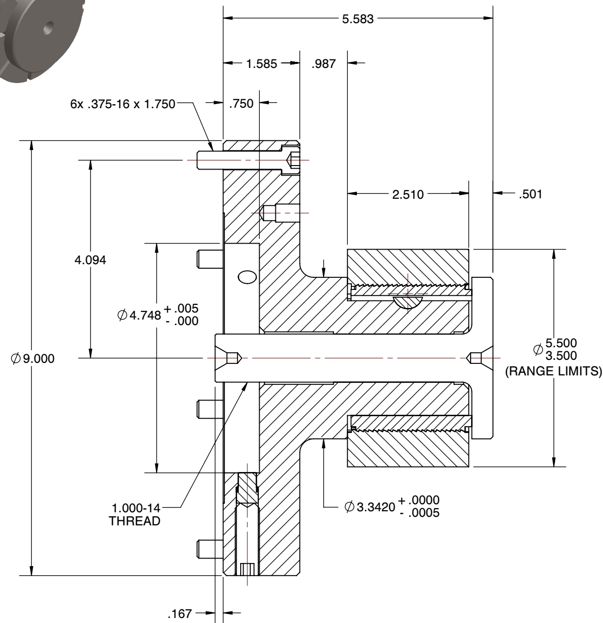
SECTION A-A
