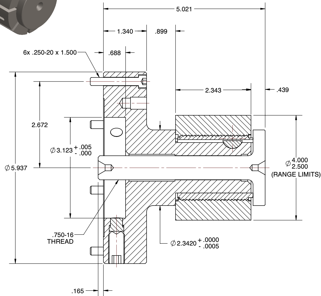
SECTION A-A
