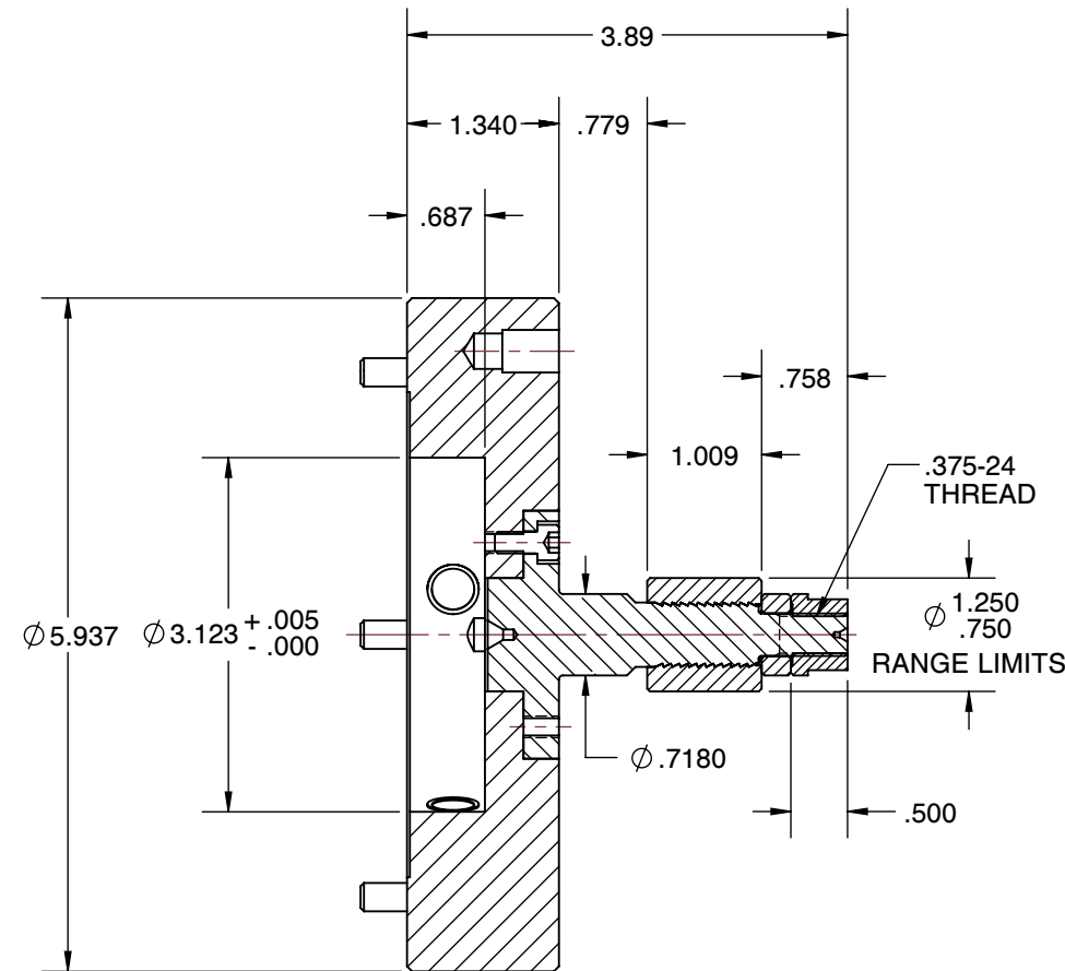
SECTION A-A
