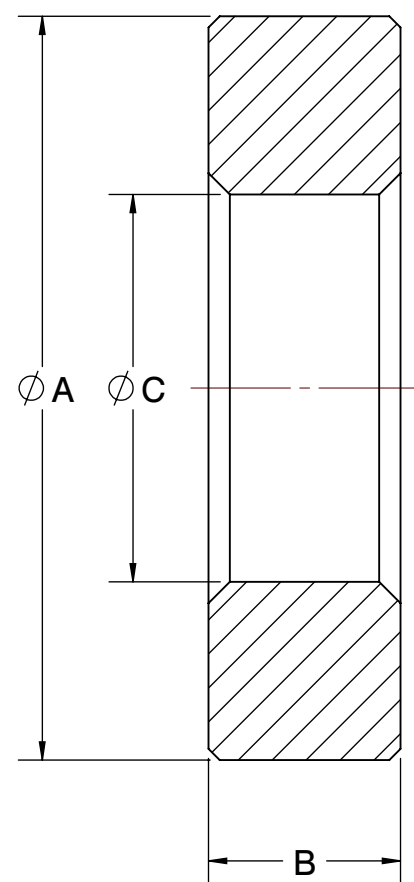
SECTION A-A
