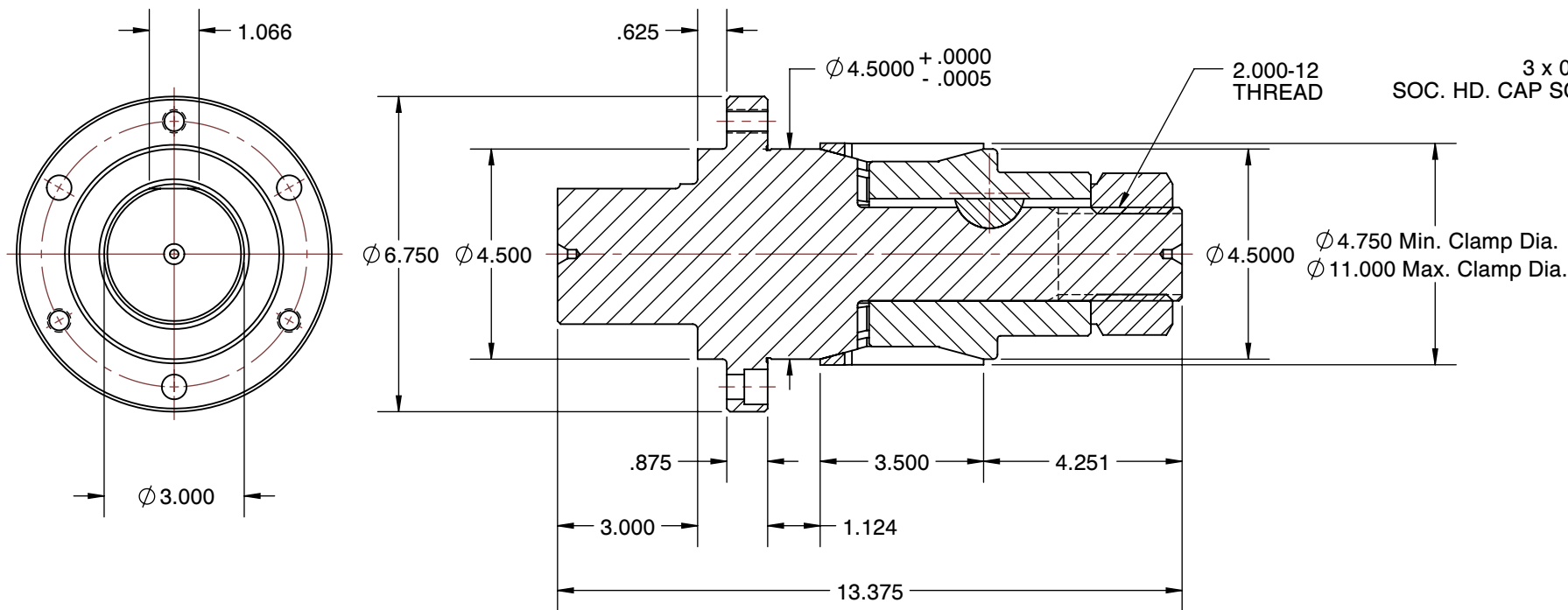
SECTION A-A
