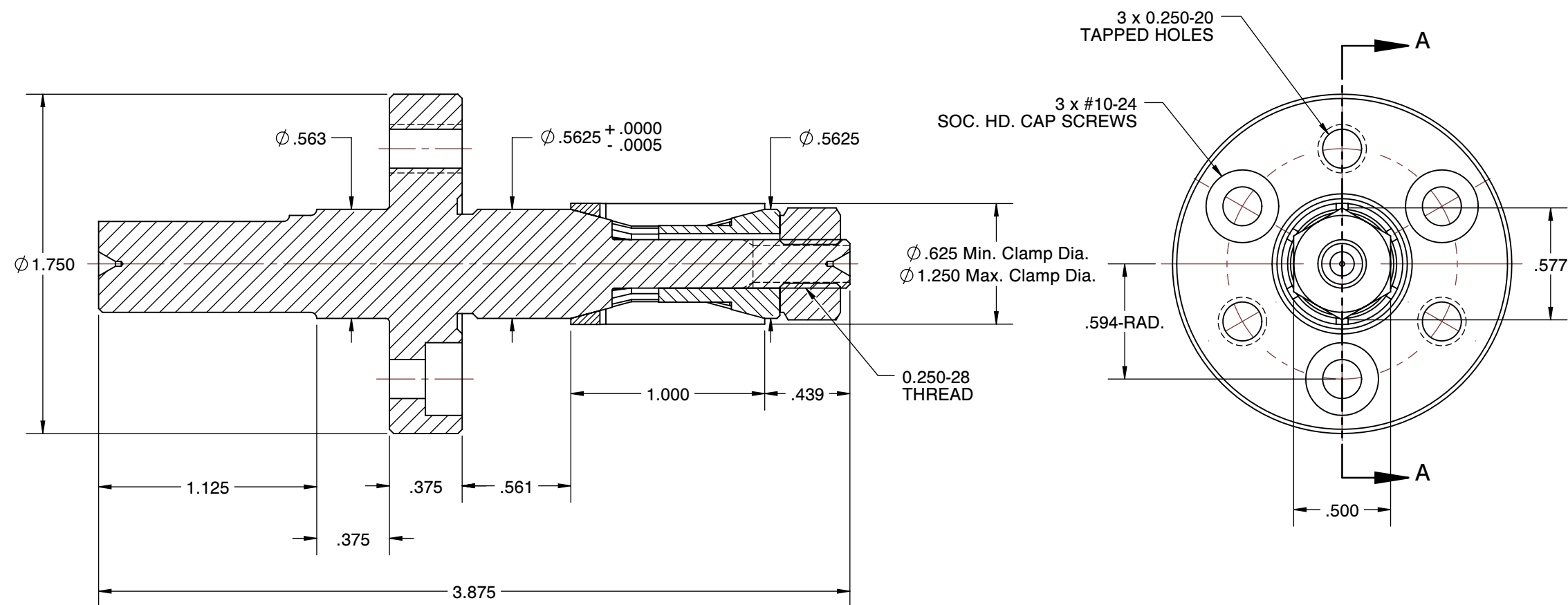
SECTION A-A
