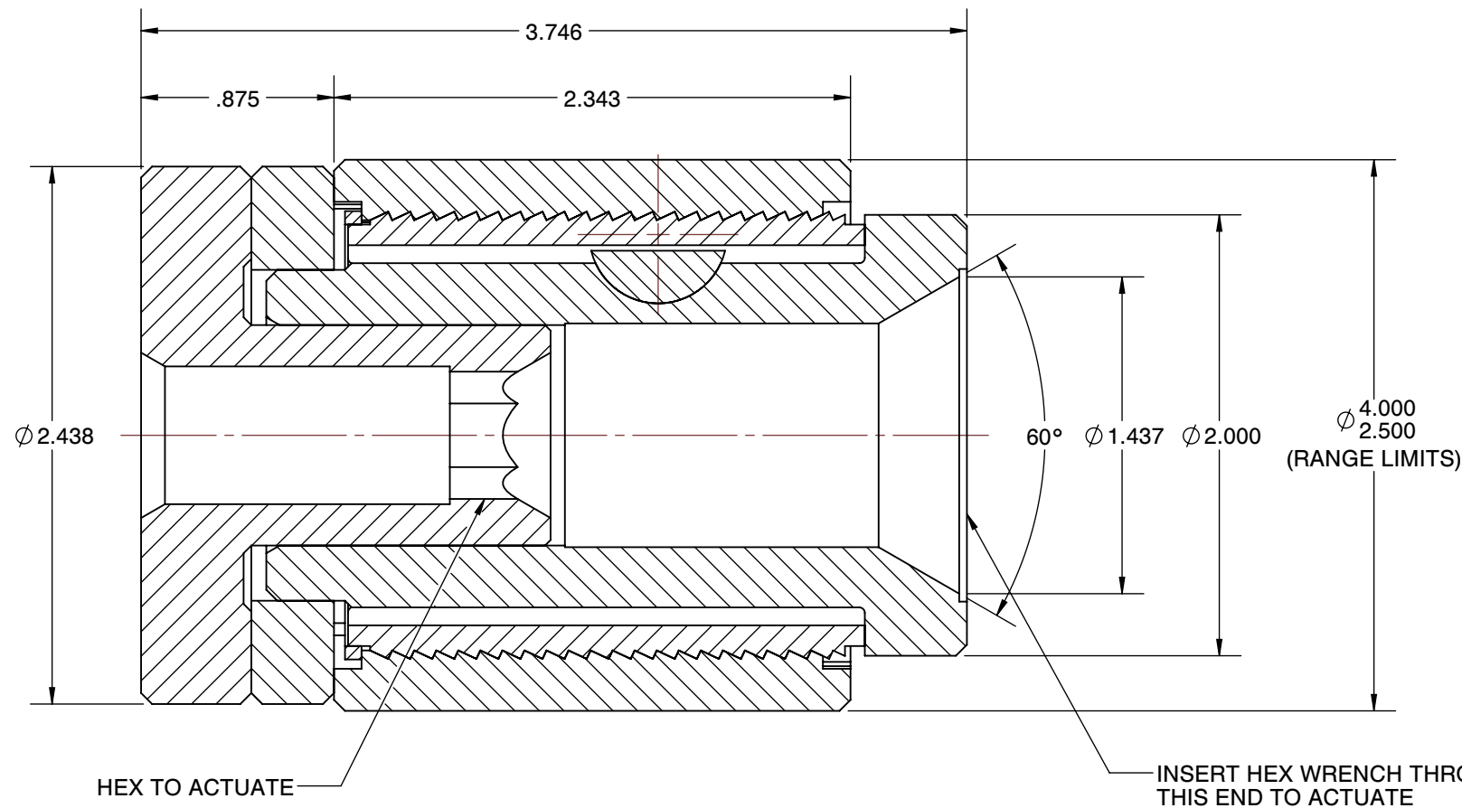
SECTION A-A
