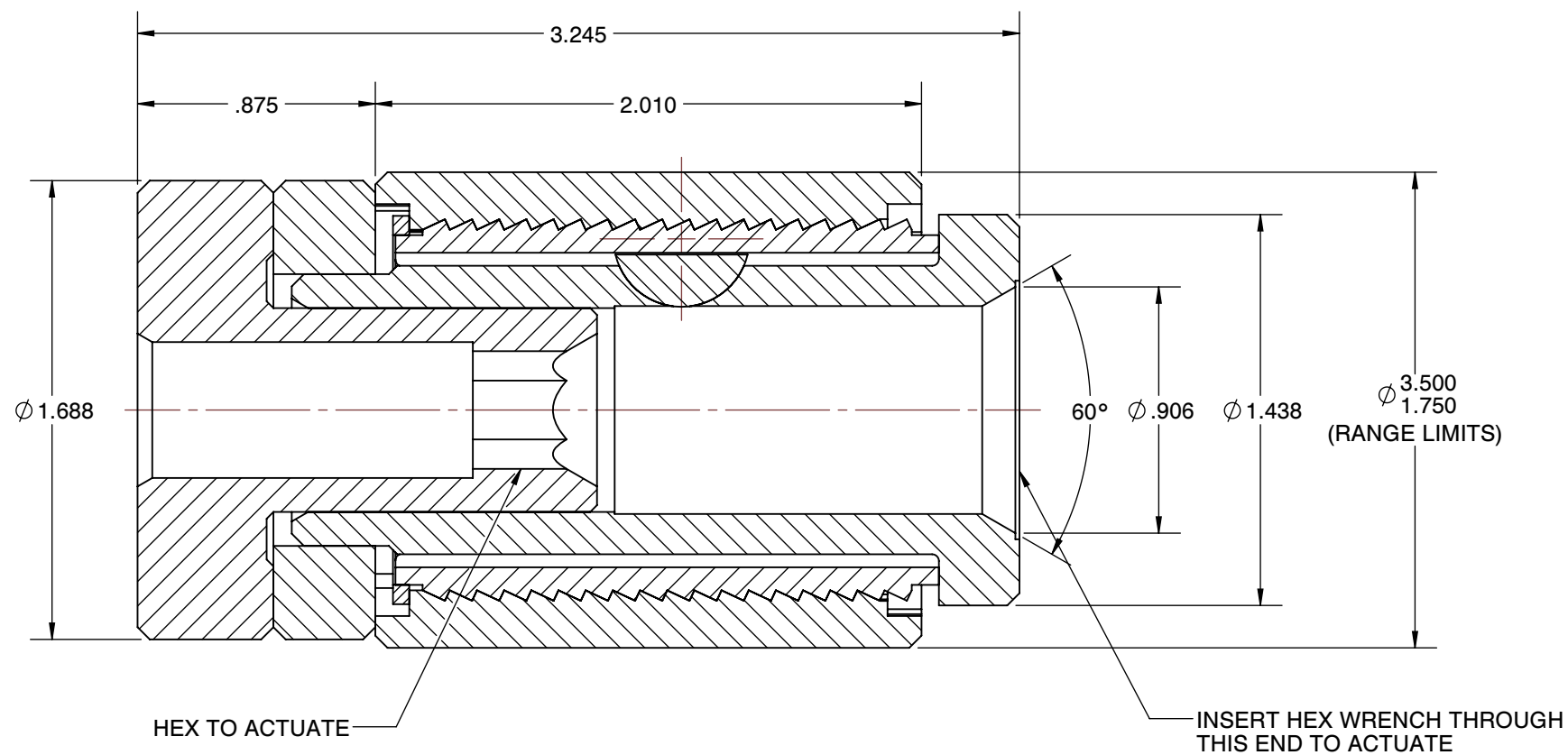
SECTION A-A
