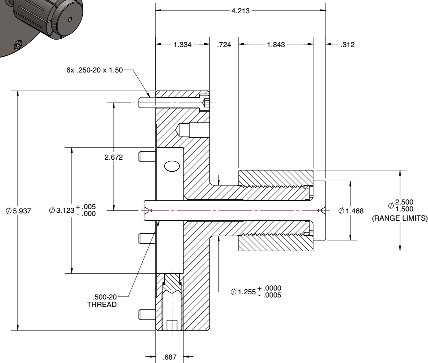
SECTION A-A
