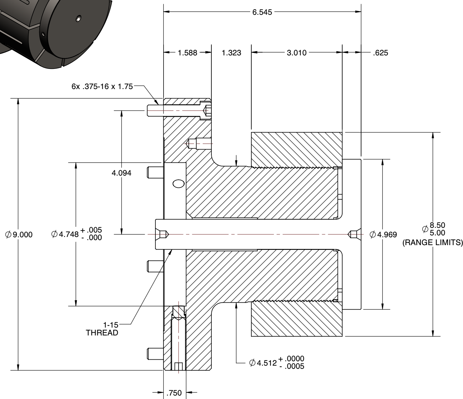
SECTION A-A
