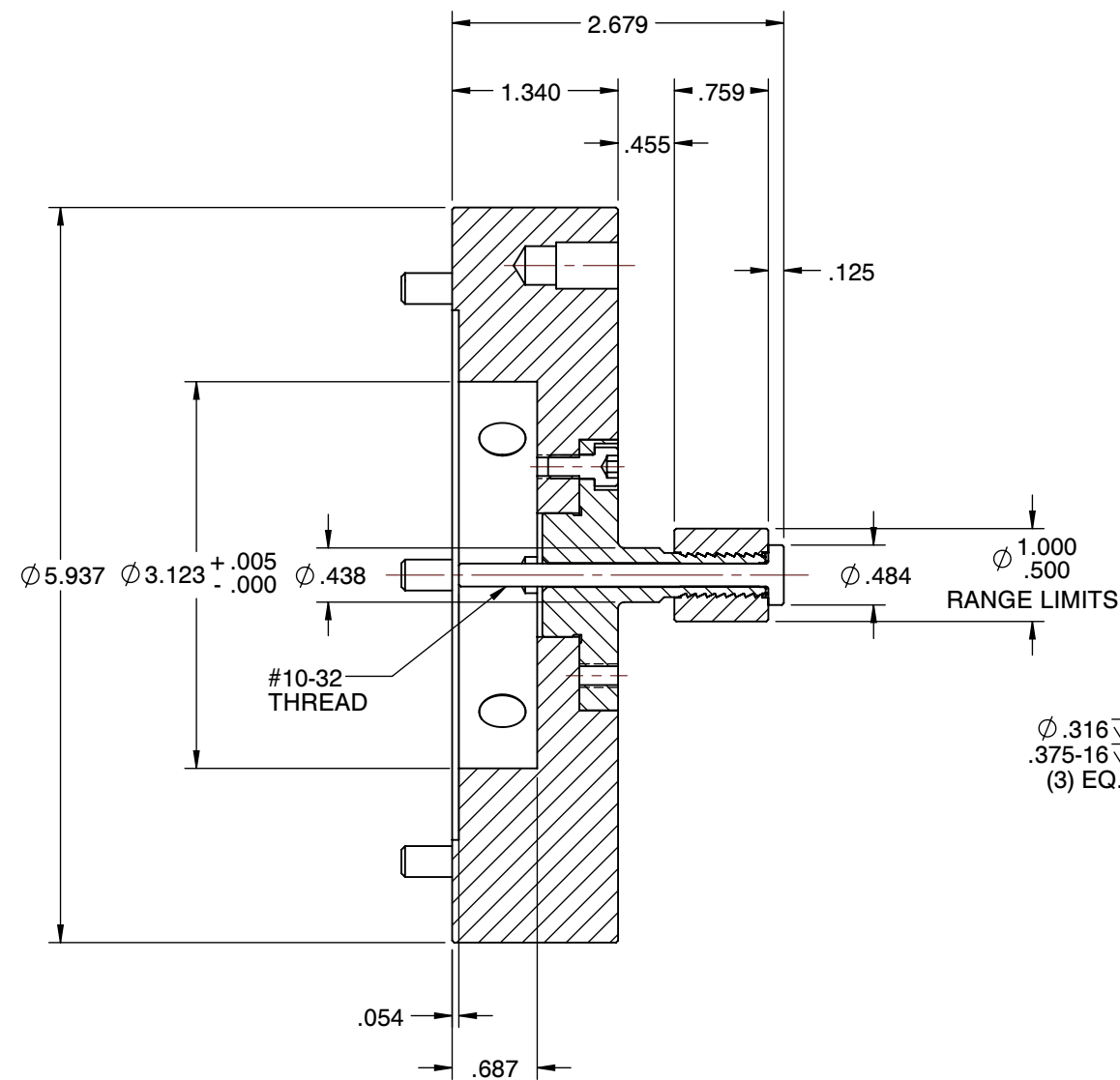
SECTION A-A
