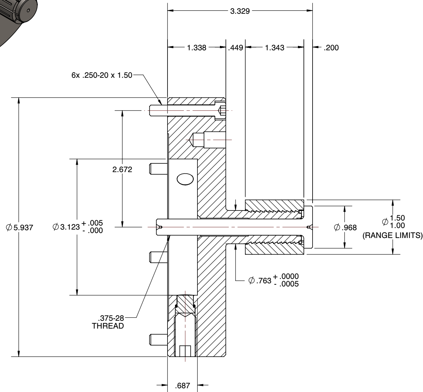
SECTION A-A
