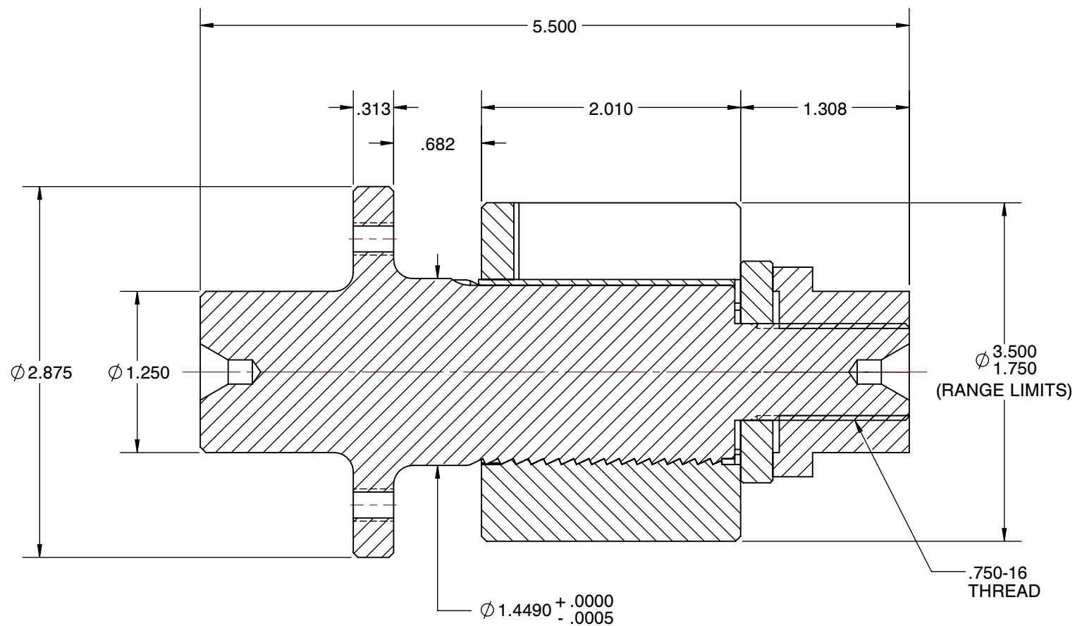
SECTION A-A
