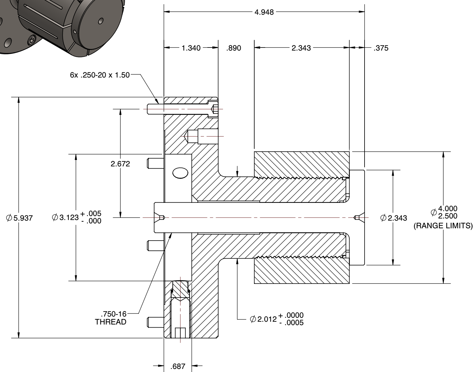
SECTION A-A
