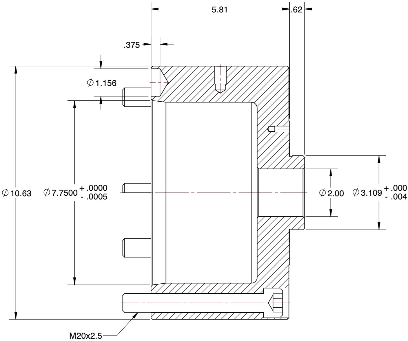
SECTION A-A
