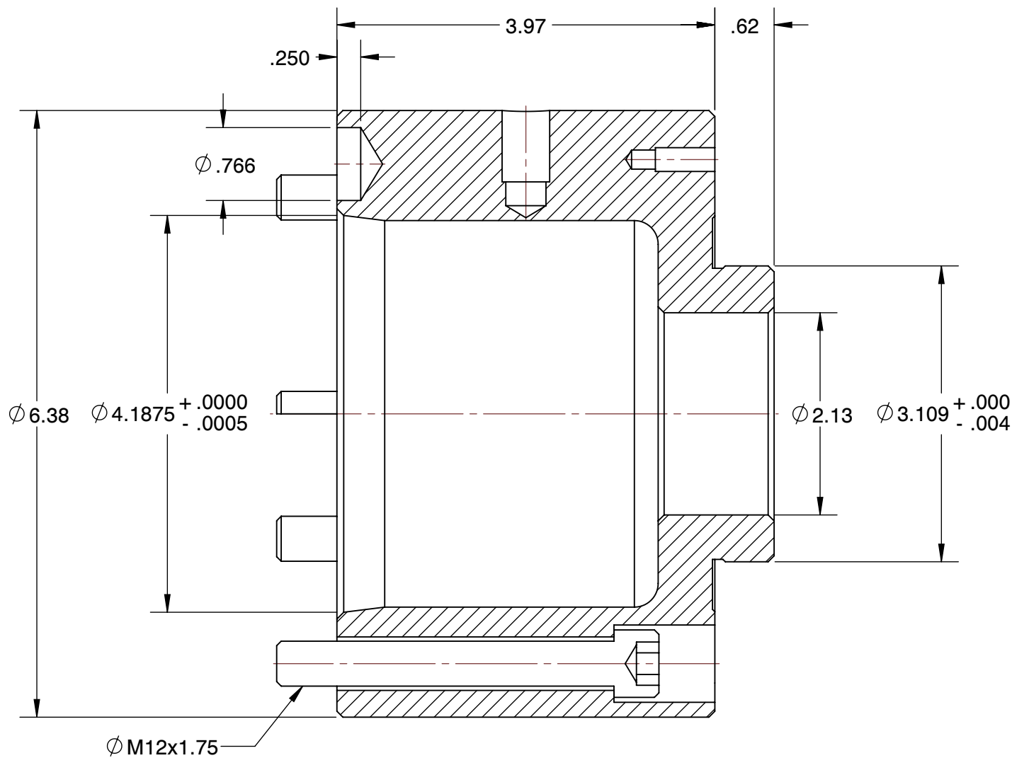
SECTION A-A
