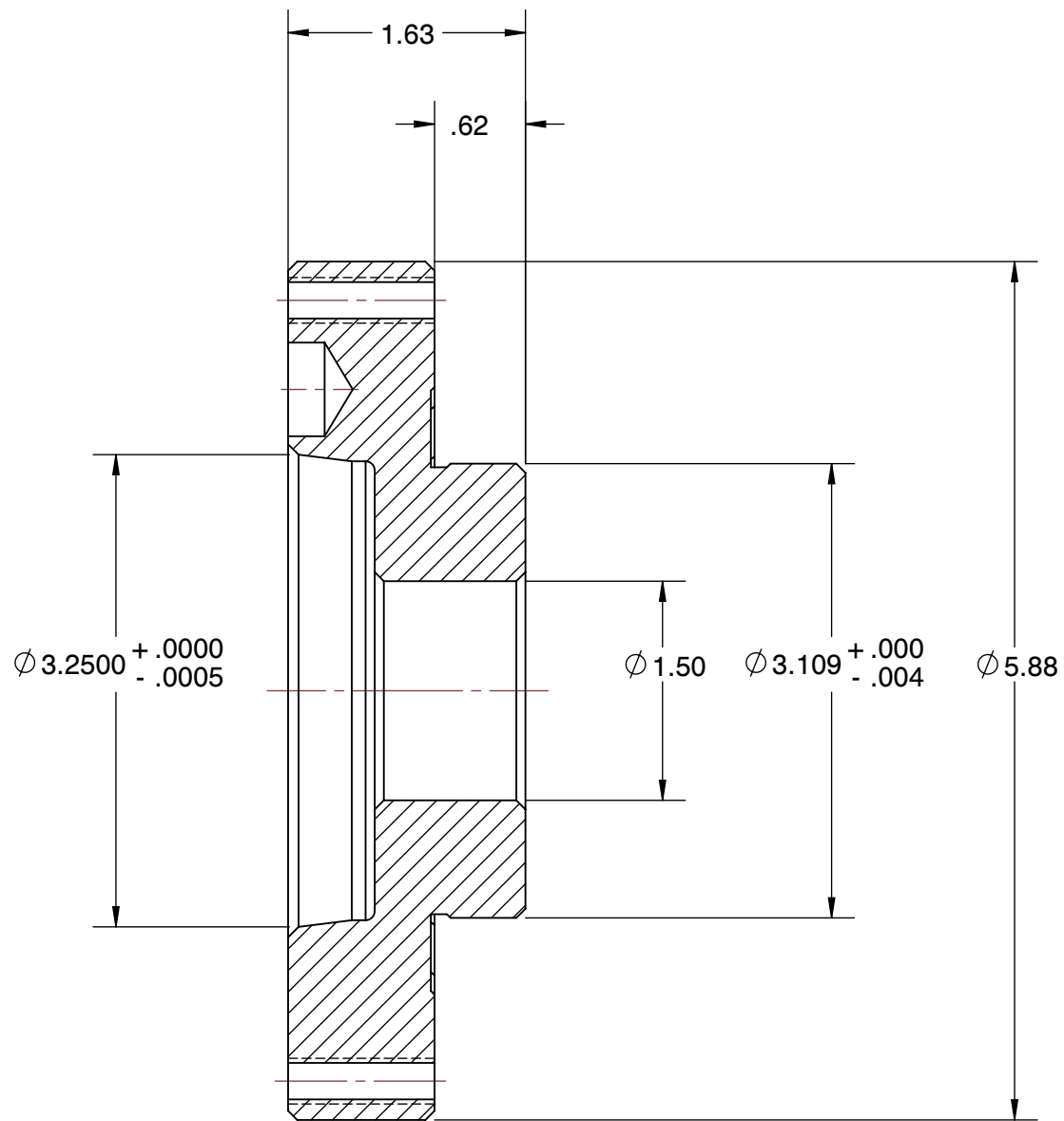
SECTION A-A
