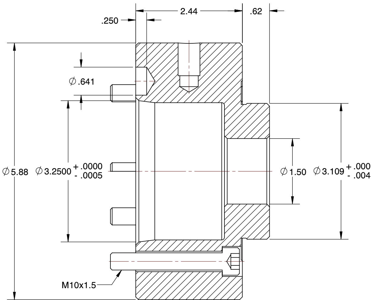
SECTION A-A
