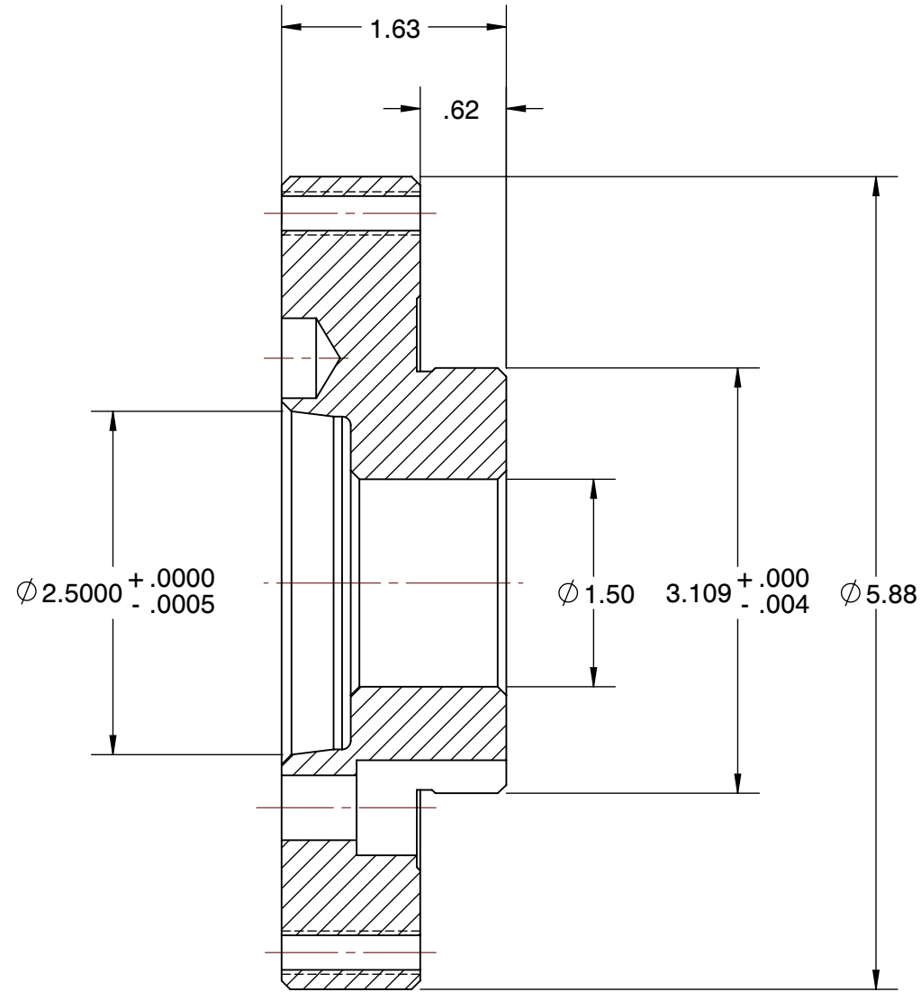
SECTION A-A
