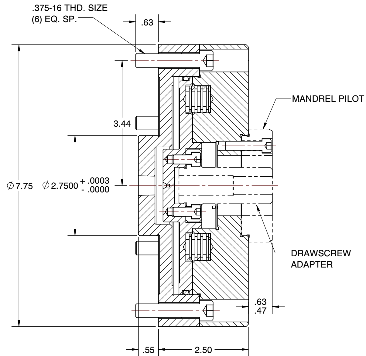
SECTION A-A
