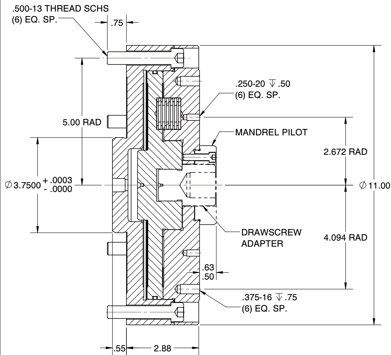
SECTION A-A
